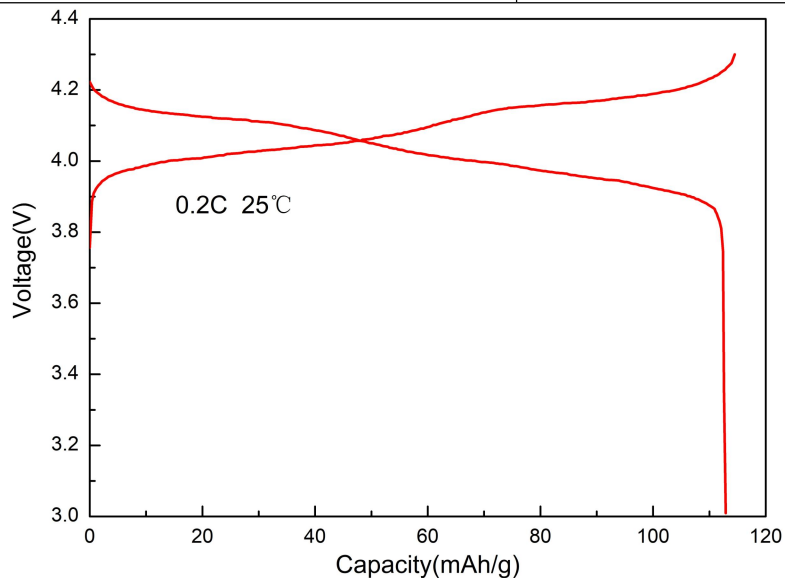
DXM-1182 充放电曲线
