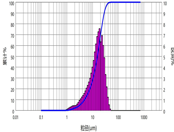
DXM-1182 激光粒度分布曲线
